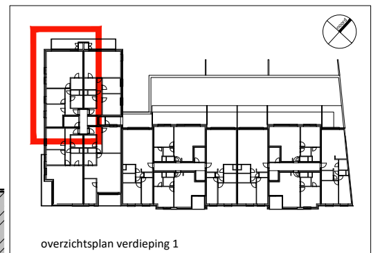
overzichtsplan verdieping 1
