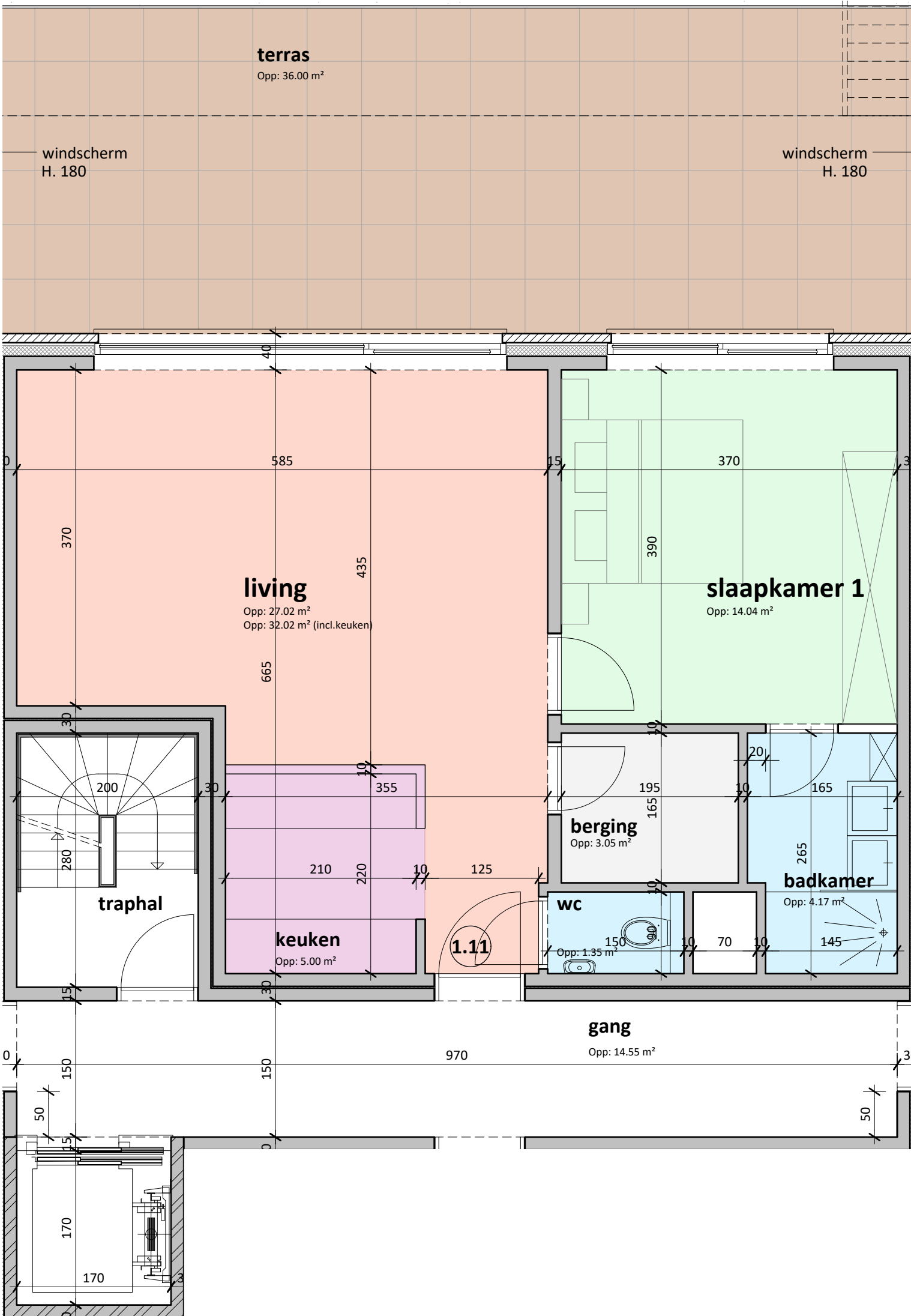
overzichtsplan verdieping 1
